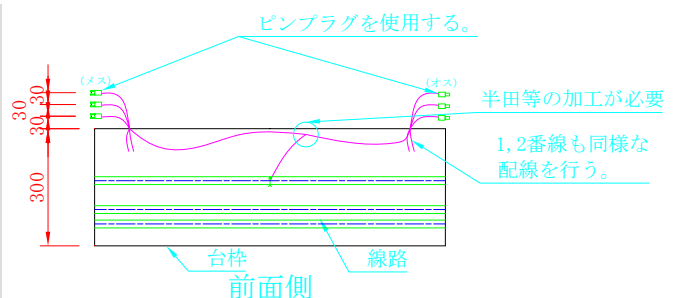
図-14 き電線の設置概要(上から透かして見た図)
