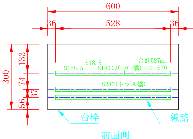
図-2 ガーター橋、トラス橋を組み込んだ線路の例
