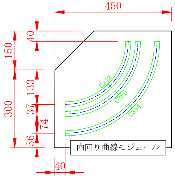
図-10 内回り曲線モジュール基本線路配置
